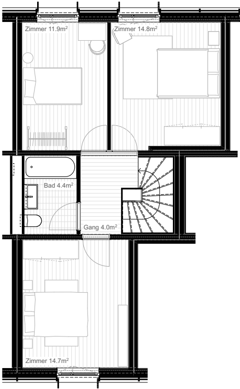
1. Obergeschoss
